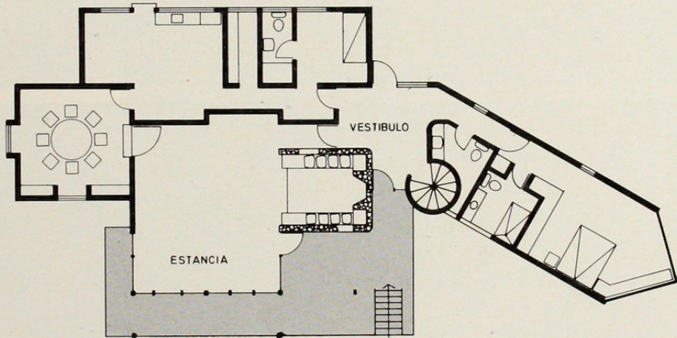
PLANTA BAJA 0 1 2 3MT
