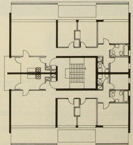
PLANTA PISO TIPO
